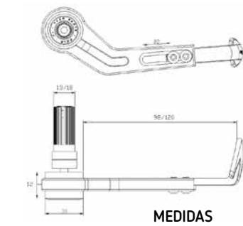
MEDIDAS
